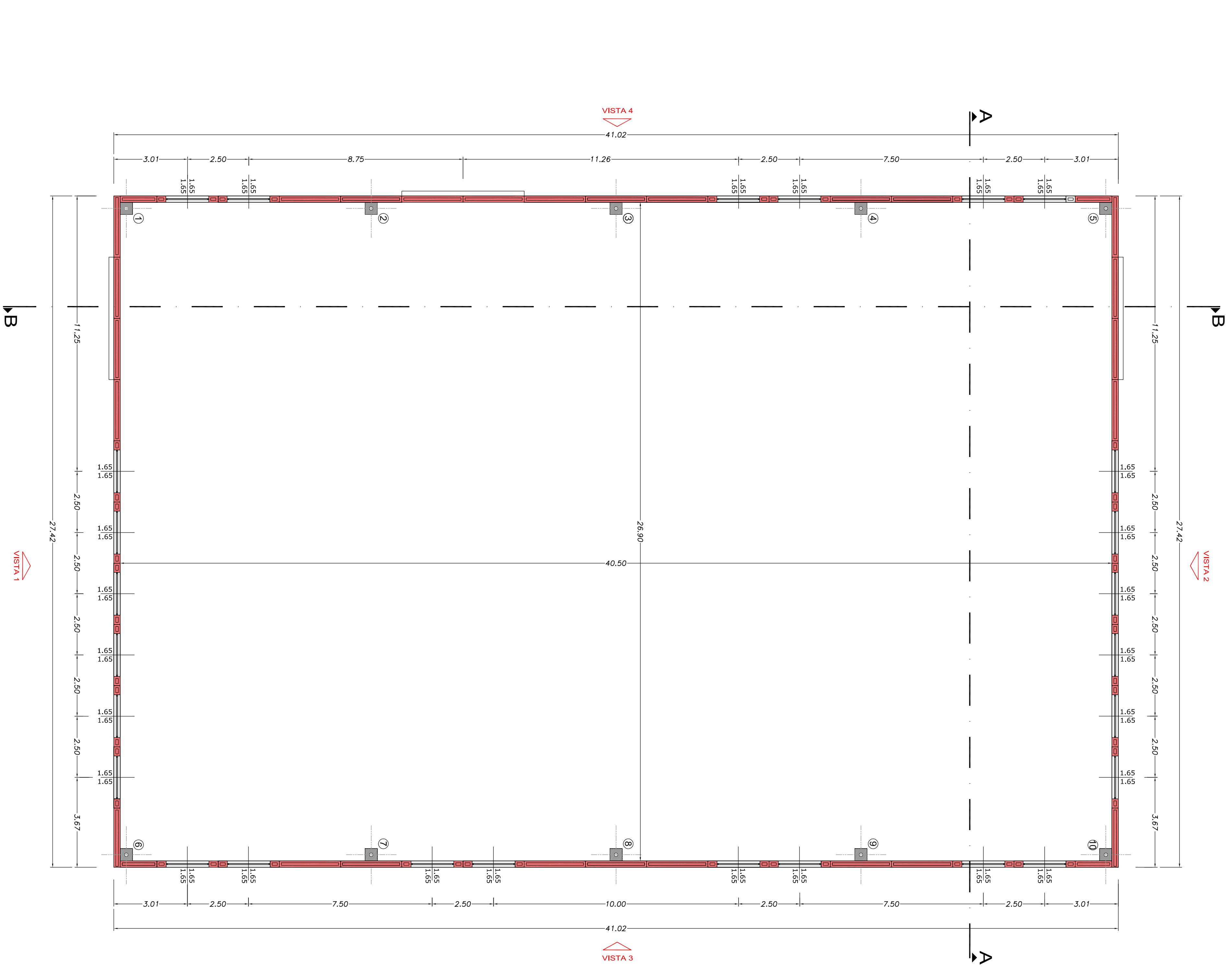
PIANTA A QUOTA 2.60
