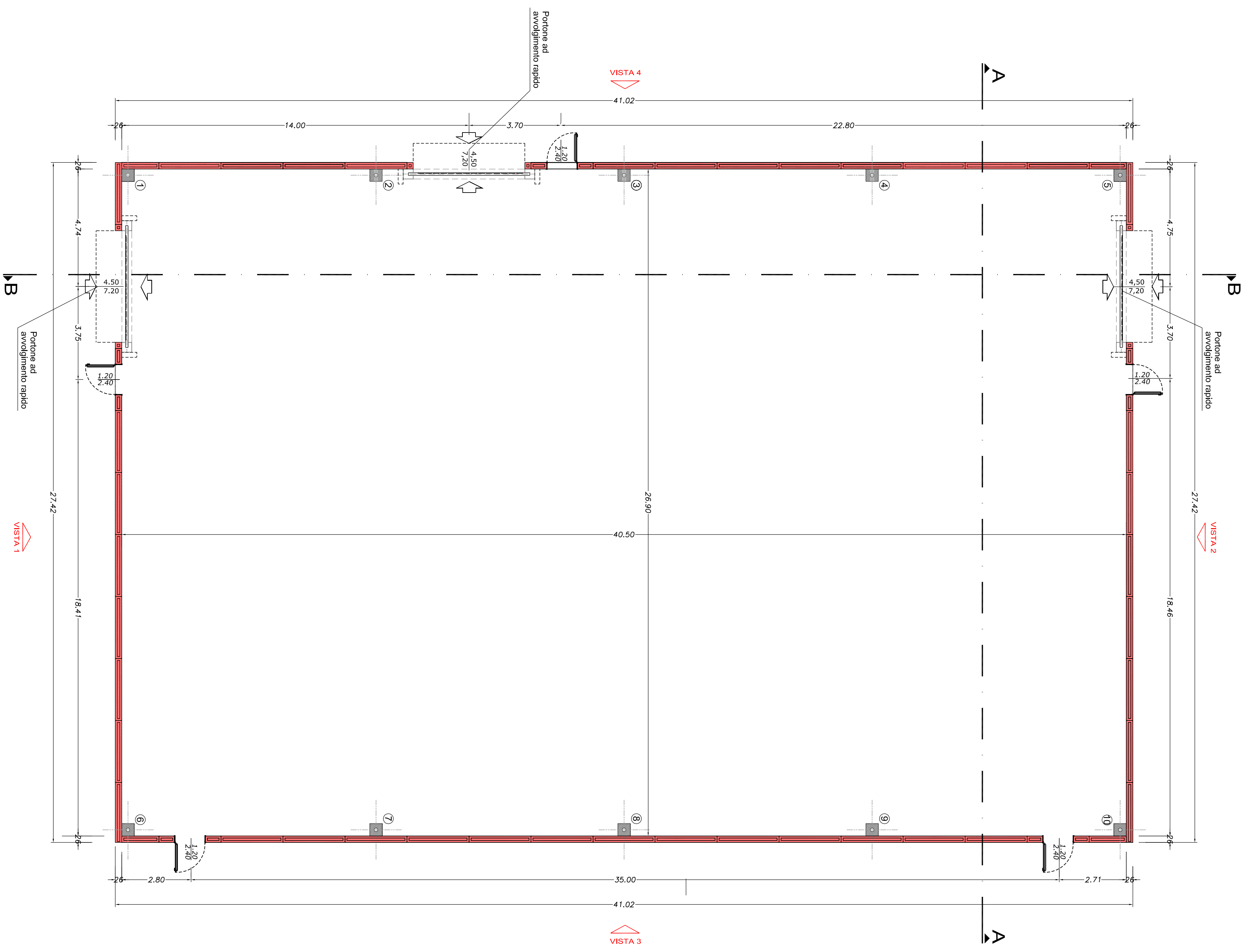
PIANTA A QUOTA 2.60
